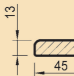
Sezione traversa
